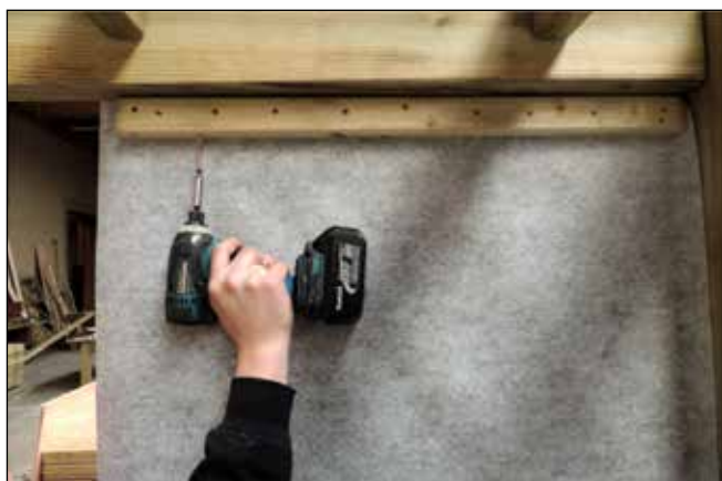
Visser le cadre de la paroi dans la poutre du dessus à l'aide de 2 vis 5x70mm
