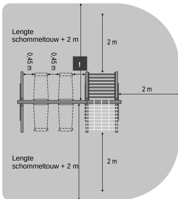
Plan met buitenafmetingen en veiligheidsafstanden voor Swing-module
